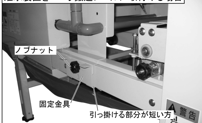
灌水装置をローラ搬送レーンに取付ける場合
