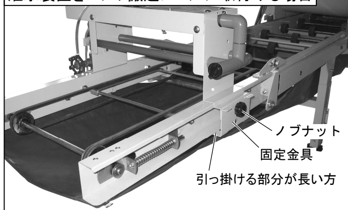
灌水装置をベルト搬送レーンに取付ける場合
